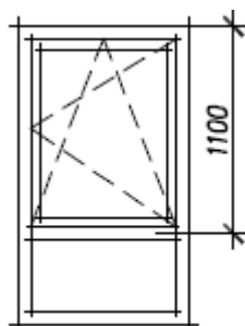
Obrázek č. 2 – Okna na severní straně restaurace „U Kopačky“
