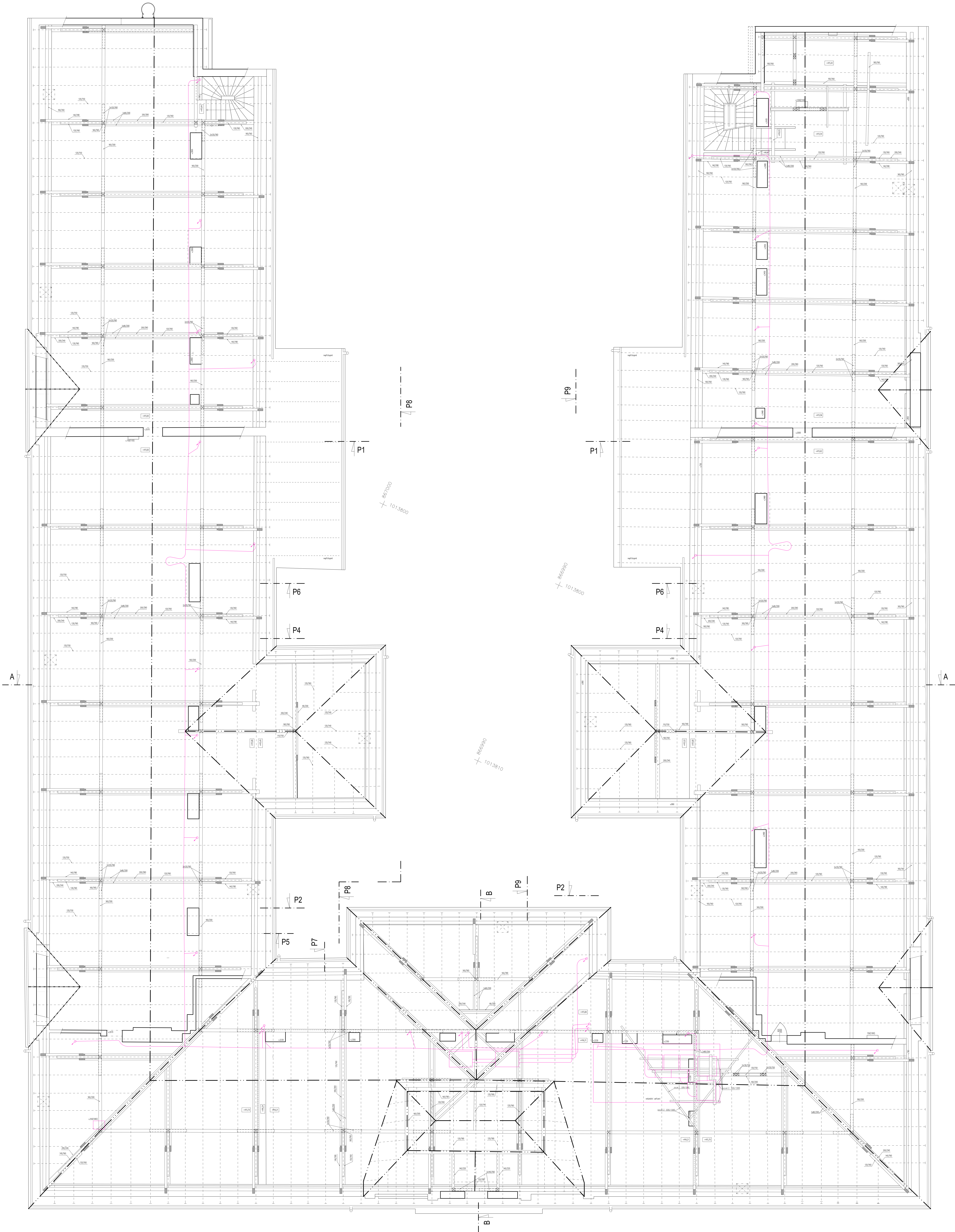
ZŠ Sokolov - krov
